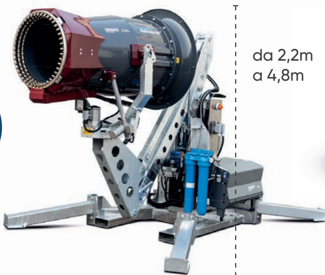
ELEFANTE 90 SU BRACCIO IDRAULICO
