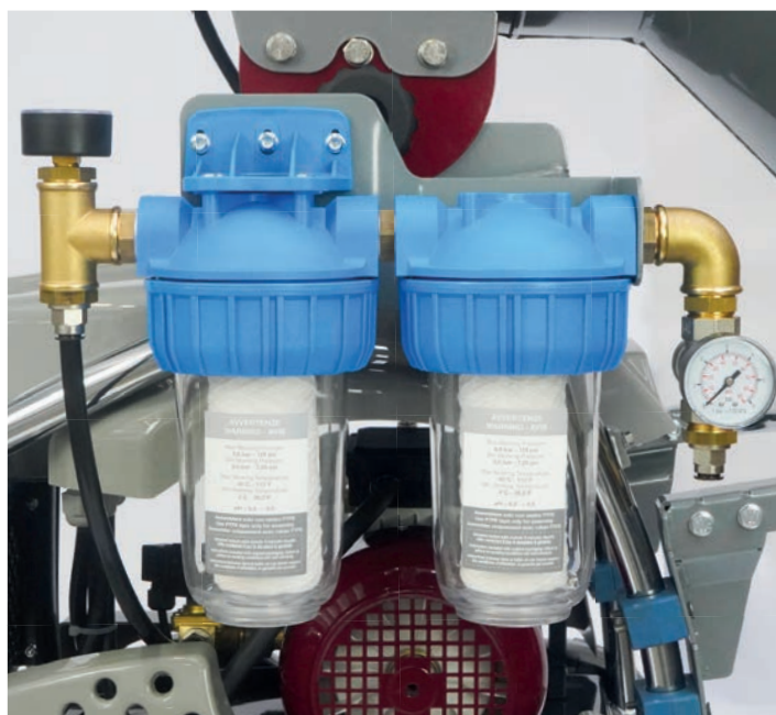
Kit ingresso acqua, livellatore di pressione e doppio filtro da 5" e 1"
