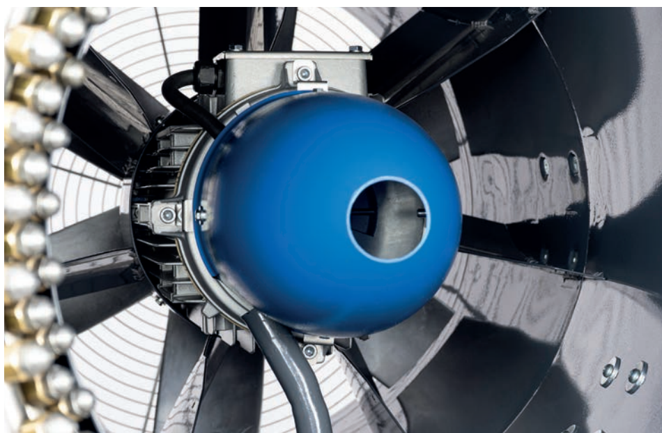
Motore ventola e configurazione dell'elica per operare a 90 metri
