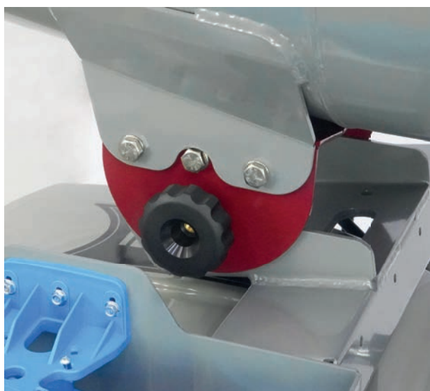
Sistema di alzo manuale semplice e robusto
